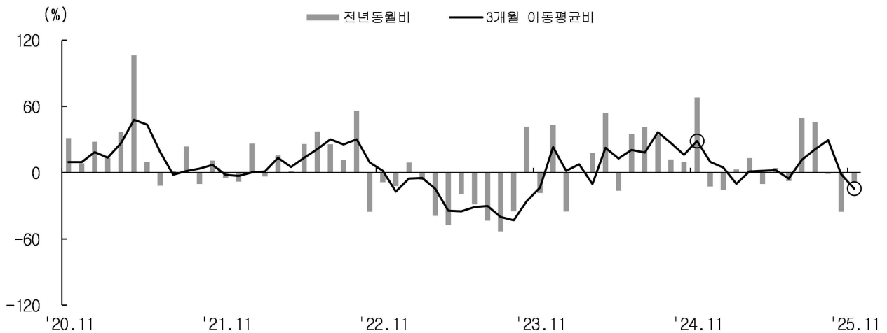
< 건설수주(전년동월비) 추이 >
