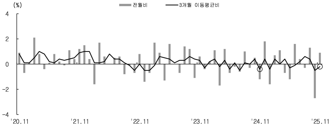
< 전산업생산지수(전월비) 추이 >
