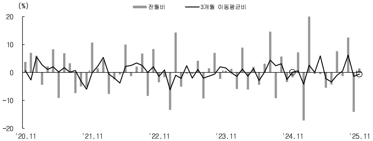
< 설비투자지수(전월비) 추이 >
