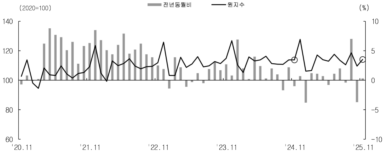
< 전산업생산지수(전년동월비) 추이 >
