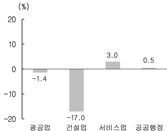
< 산업별 전년동월비 >
