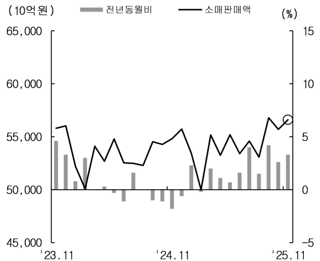
< 소매판매액(전년동월비) 추이 >
