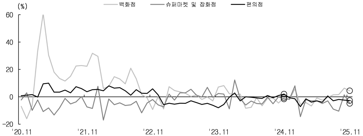
< 소매업태별지수(전년동월비) 추이1 >
