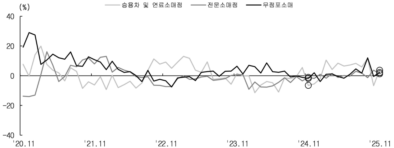
< 소매업태별지수(전년동월비) 추이2 >
